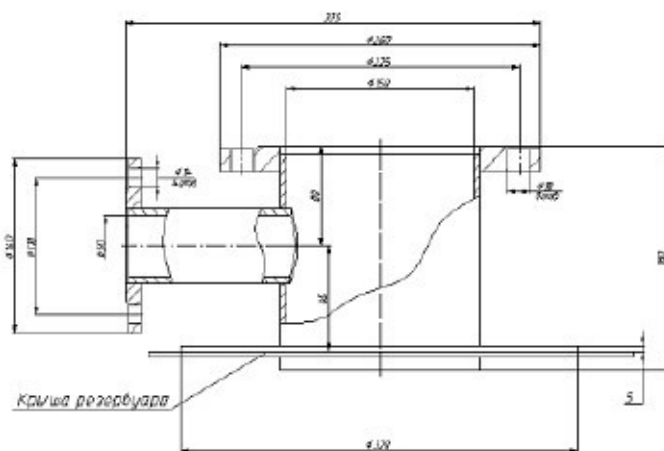
Общий вид патрубка замерного люка ПЗЛ-150
